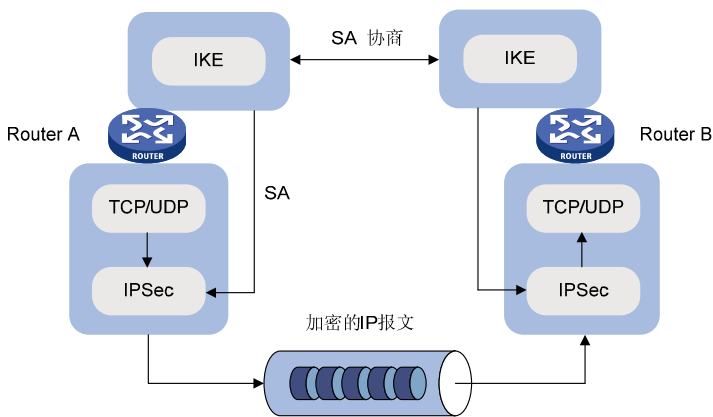
图7-5 IPSec 与 IKE 的关系图
