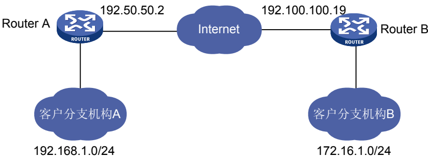
图7-3 组网示意图
